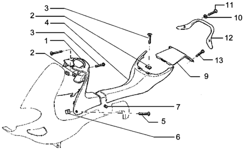
Verkleidung Fußraum
