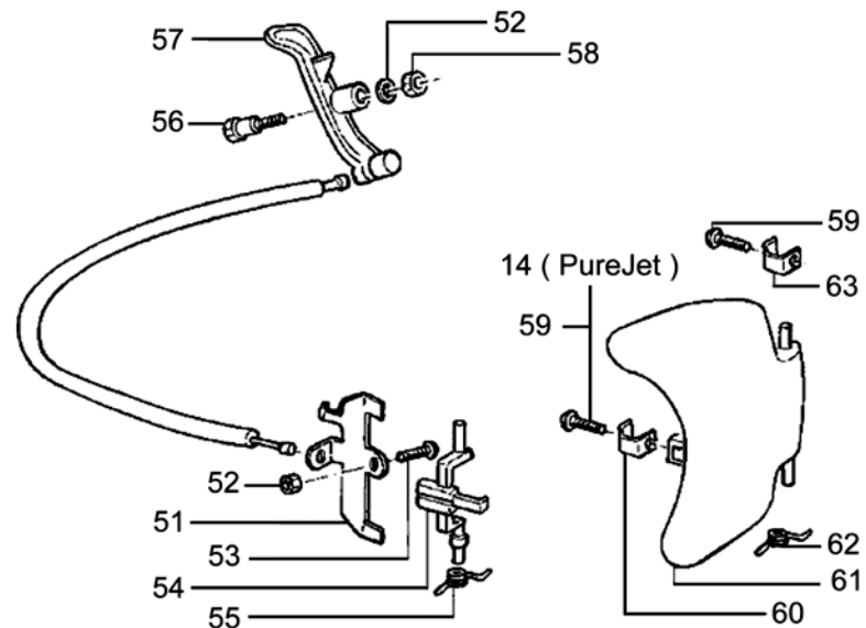
Tankklappe / Lenkradschloß
