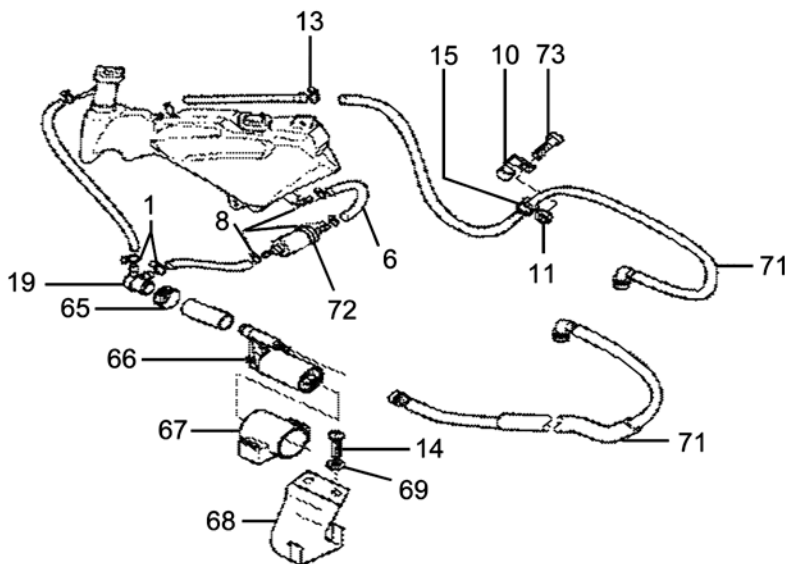
Kraftstoffanlage PureJet
