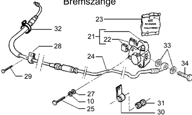
Bremszange
