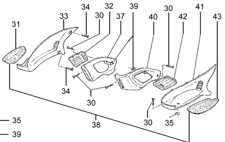
Verkleidung Fußraum
