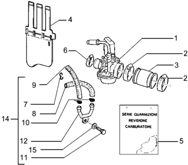
Vergaser / Drosselkörper
