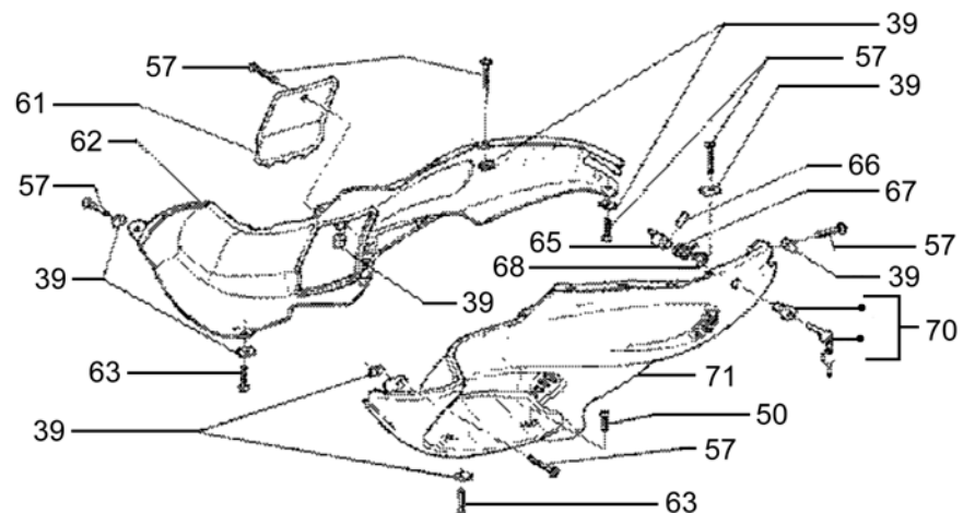
Verkleidung seitlich
