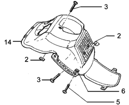
Verkleidung unten
