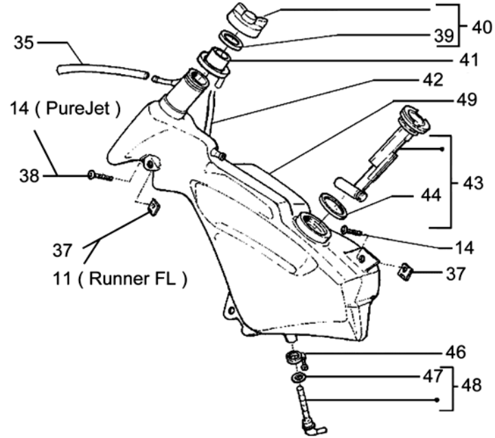
Benzintank
