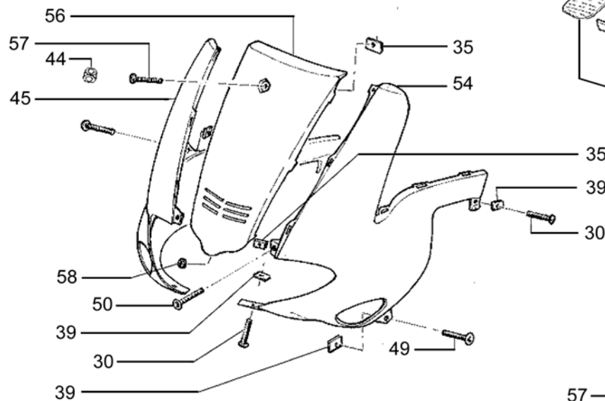
Verkleidung vorne
