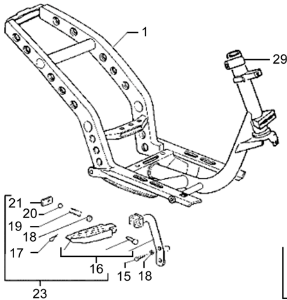
Rahmen / Ständer
